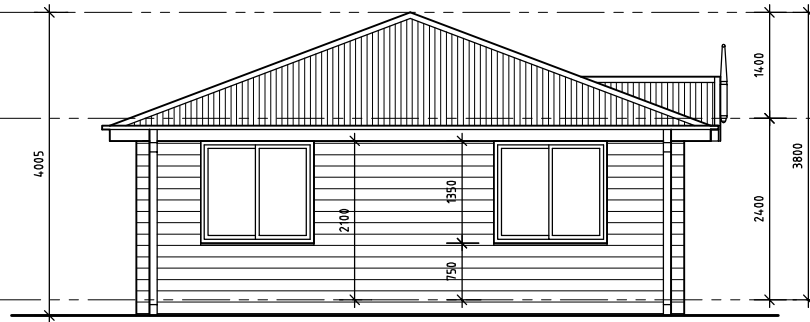
B SIDE ELEVATION - 1:50
