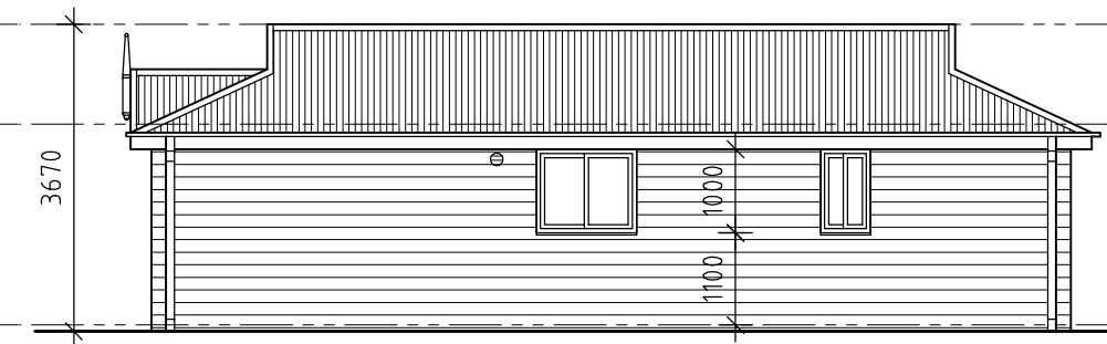
D SIDE ELEVATION - 1:50
