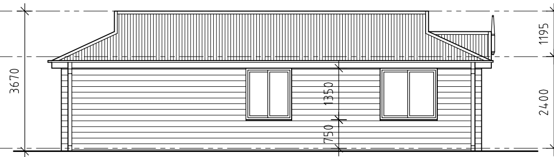
B SIDE ELEVATION - 1:50
