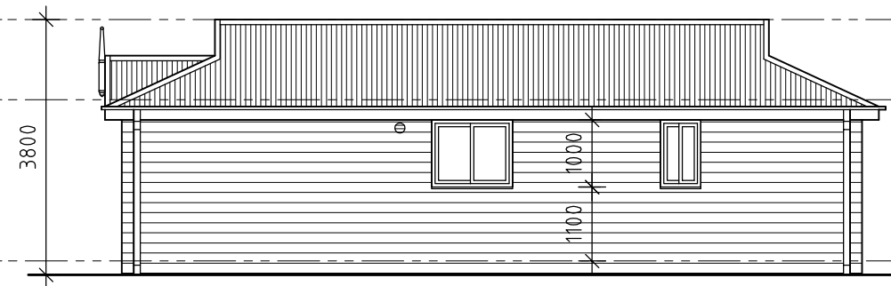
D SIDE ELEVATION - 1:50
